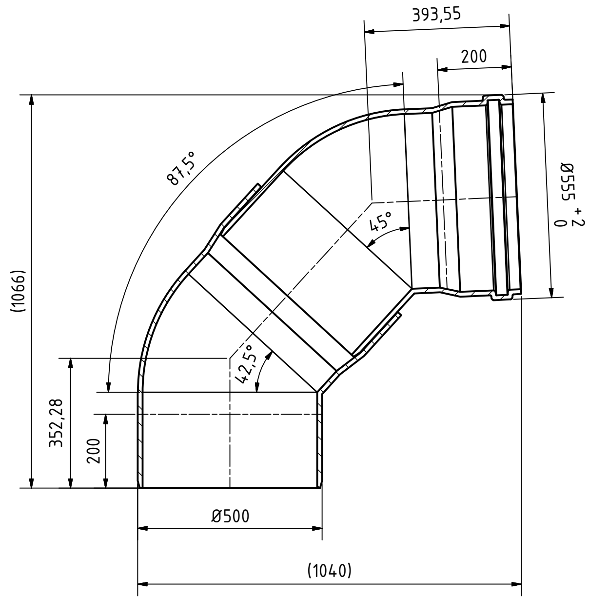
A-A ( 1 : 10 )
