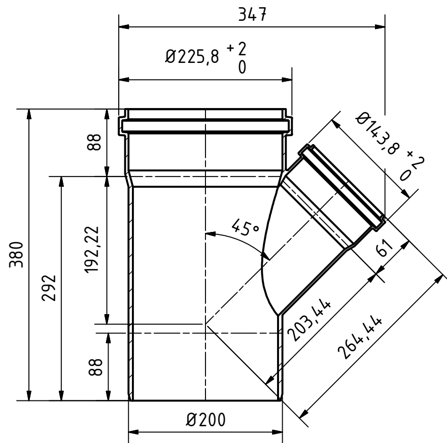
A-A ( 1 : 5 )
