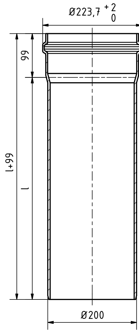
A-A ( 1 : 5 )
