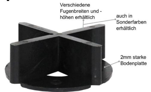
Abbildung 1: Fugenkreuz mit Bodenplatte, Farbe: schwarz
