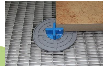
Abbildung 4: FK-B mit VP-GKU auf Gitterrost verlegt
